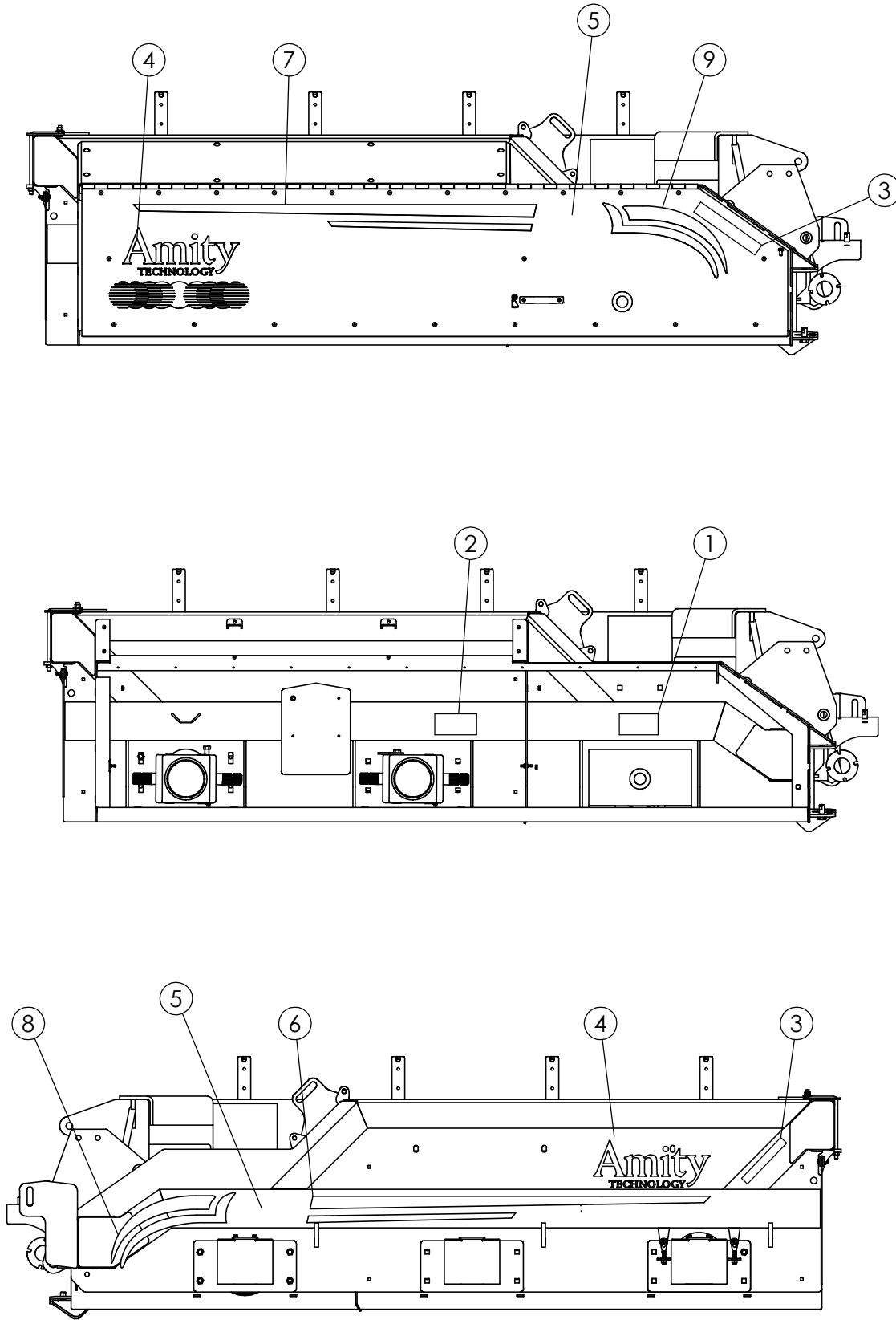
LEFT SIDE
