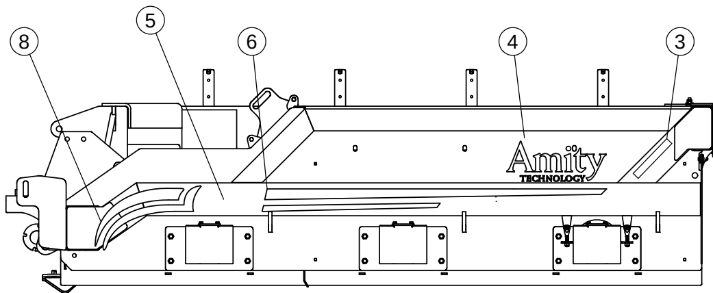
LEFT SIDE
