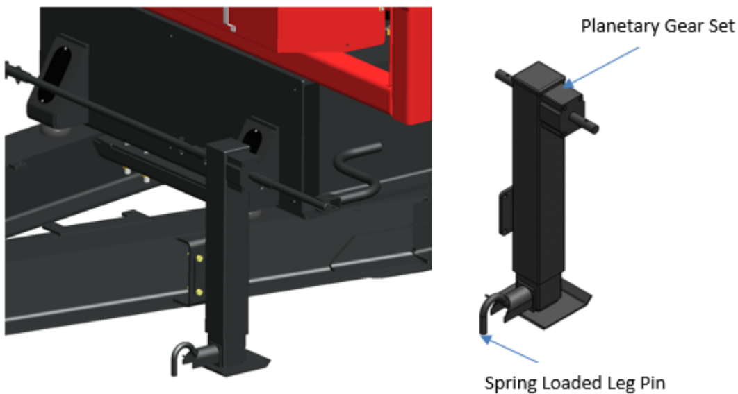
Рисунок 6-9: Стенды
