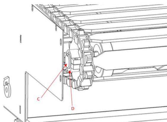
Рисунок 7-11b: Шфт пола
